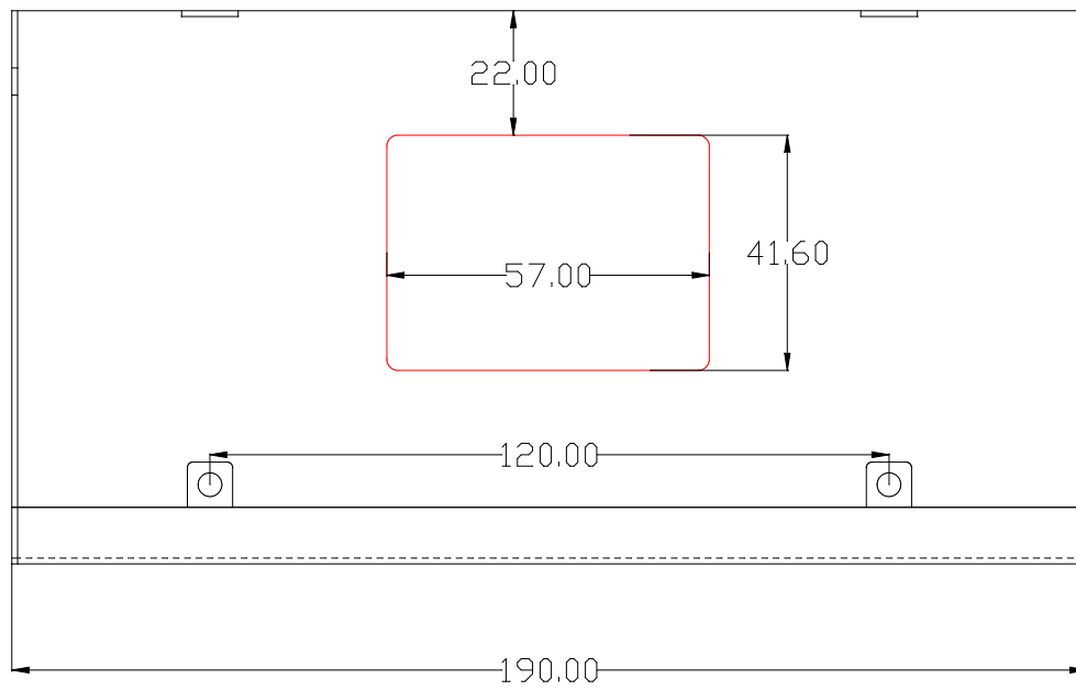
俯视图:
